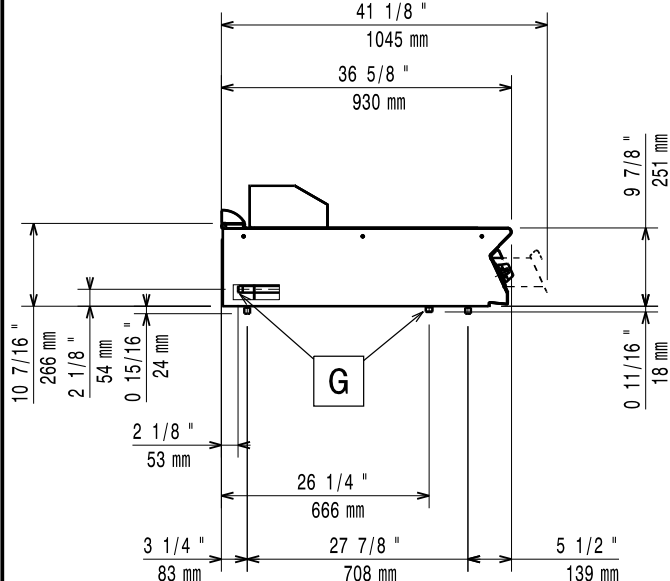
Oldalnézet
